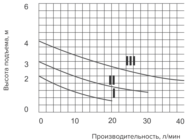
Рисунок 2 — График соотношения высоты подъема и производительности для насоса циркуляционного I-TECH 25/4/180
