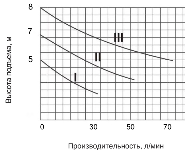
Рисунок 4 - График соотношения напора и производительности для насоса циркуляционного I-TECH 25/8/180
